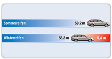
Bremsvergleich Sommer-/Winterreifen bei Nässe unter +7°C (Reifen- und Fahrzeugspezifische Abweichungen möglich)
